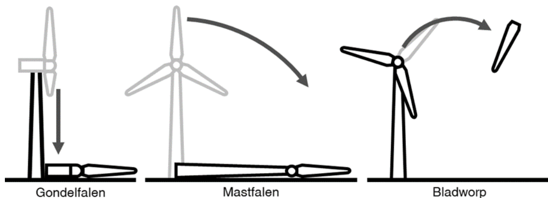
Figuur 7 Mogelijke faalscenario's van een windturbine, de effectafstand is de maximale afstand tot waar een scenario een effect heeft
